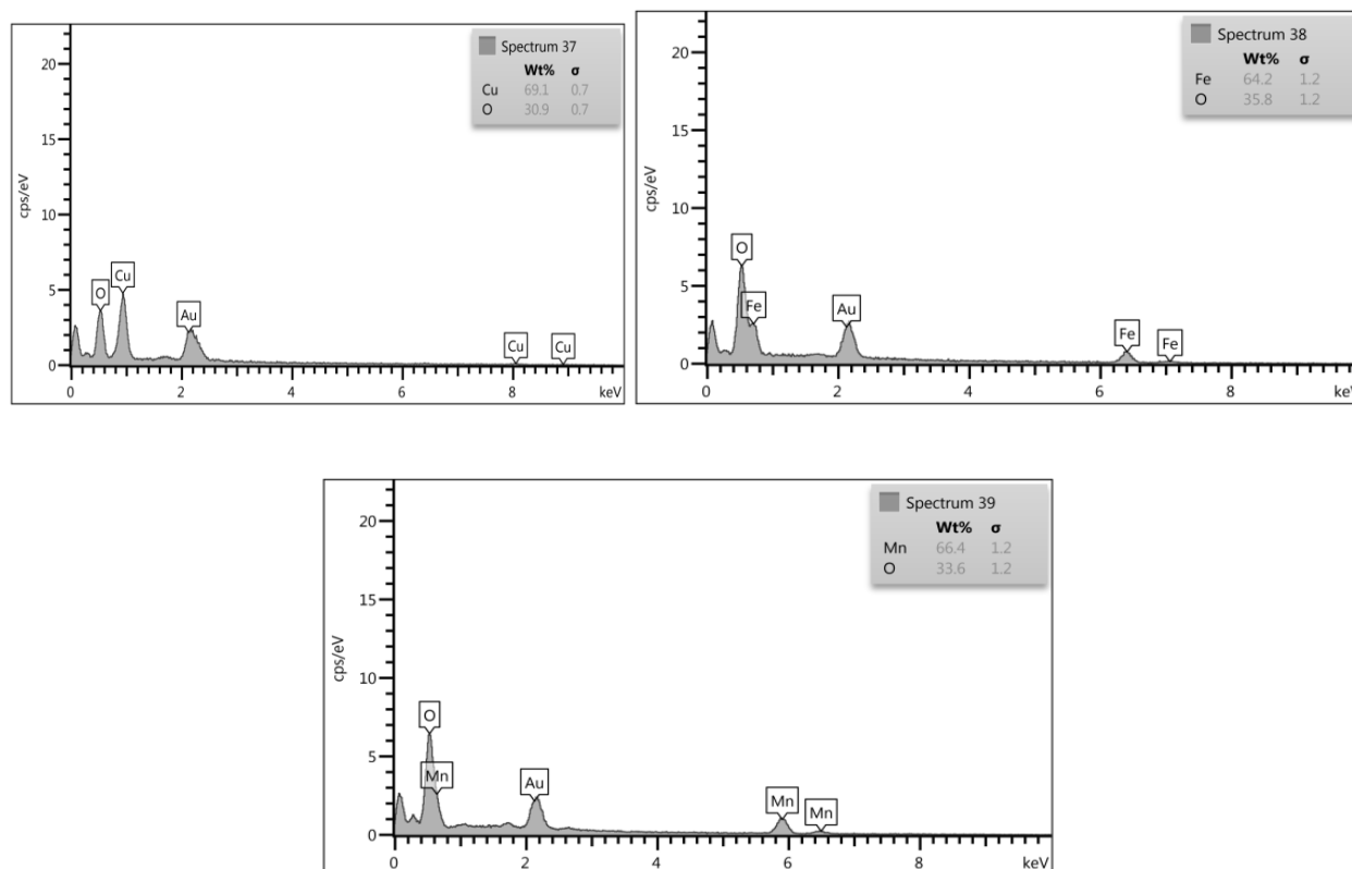
شکل ۳. طیف EDS (a) بورات مس، (b) بورات آهن، و (c) بورات منگنز
