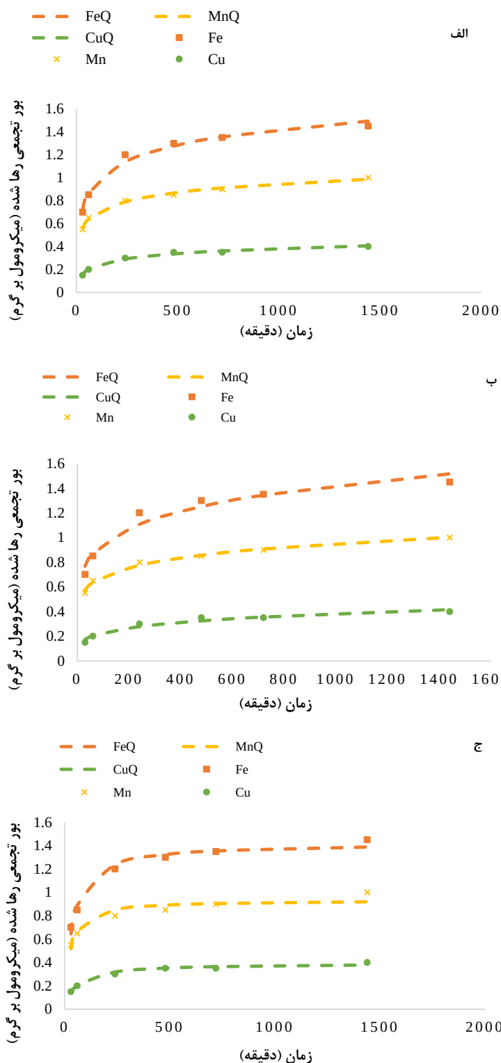
شکل ۴. رهاسازی وابسته به زمان بُور از نانو ترکیبات بُورات مس، بُورات آهن و بُورات منگنز. خطوط نقطه چین، برازش مدل الویچ (الف)، مدل تابع توانی (ب) و مدل شبه رده دوم (ج) بر داده‌های سینتیکی را نشان می‌دهد.
