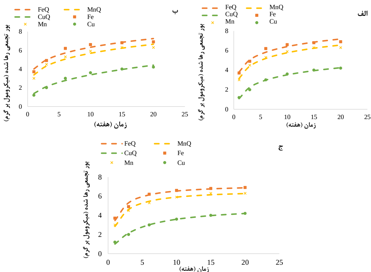
شکل ۵. رها سازی وابسته به زمان بور از نانو ترکیبات بورات مس، بورات آهن و بورات منگنز در خاک. خطوط نقطه چین، برازش مدل الوویچ (الف)، مدل تابع توانی (ب) و مدل شبه رده دوم (ج) بر داده‌های سینتیکی را نشان می‌دهد.
