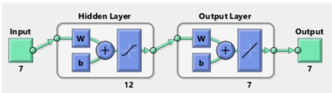
شکل ۷. ساختار شبکه عصبی بهینه در تشخیص درصدهای مختلف K_2O بر اساس ویژگی‌های کارا
