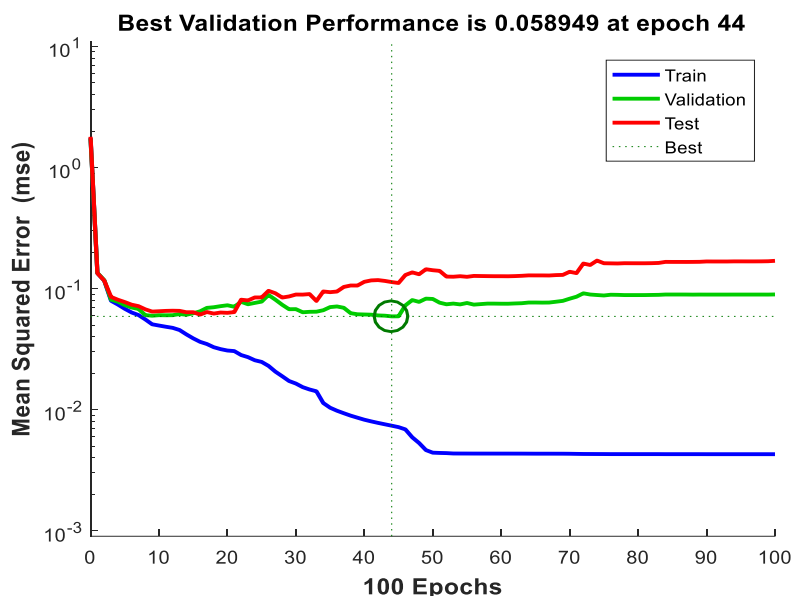
شکل ۸. نمودار عملکرد شبکه عصبی مصنوعی بهینه در تشخیص درصدهای مختلف K_2O بر اساس ویژگی‌های کارا
