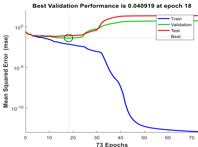
شکل ۴. نمودار عملکرد شبکه عصبی مصنوعی در مرحله اعتبارسنجی در تشخیص درصد‌های مختلف K_2O بر اساس تمام ویژگی‌های استخراج شده
