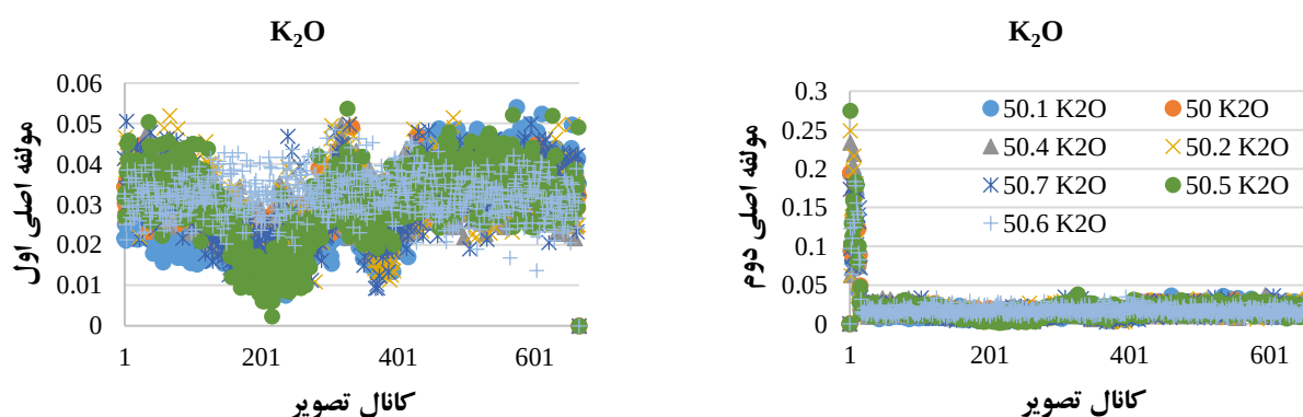
شکل ۲. نمودار مولفه‌های اصلی اول و دوم کود پتاس با سطوح مختلف اکسید پتاسیم
