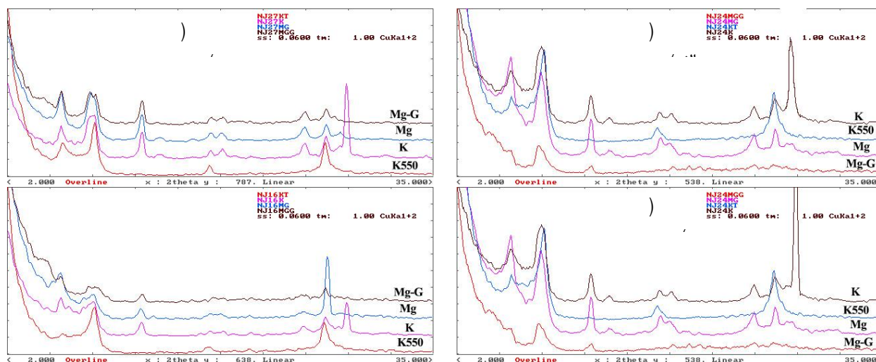
شکل ۱. نمودار پراش پرتو ایکس مربوط به ذرات کوچکتر از ۰/۰۰۲ میلی‌متر خاک‌های ۱ (الف)، ۲ (ب)، ۳ (ج) و ۴ (د)
