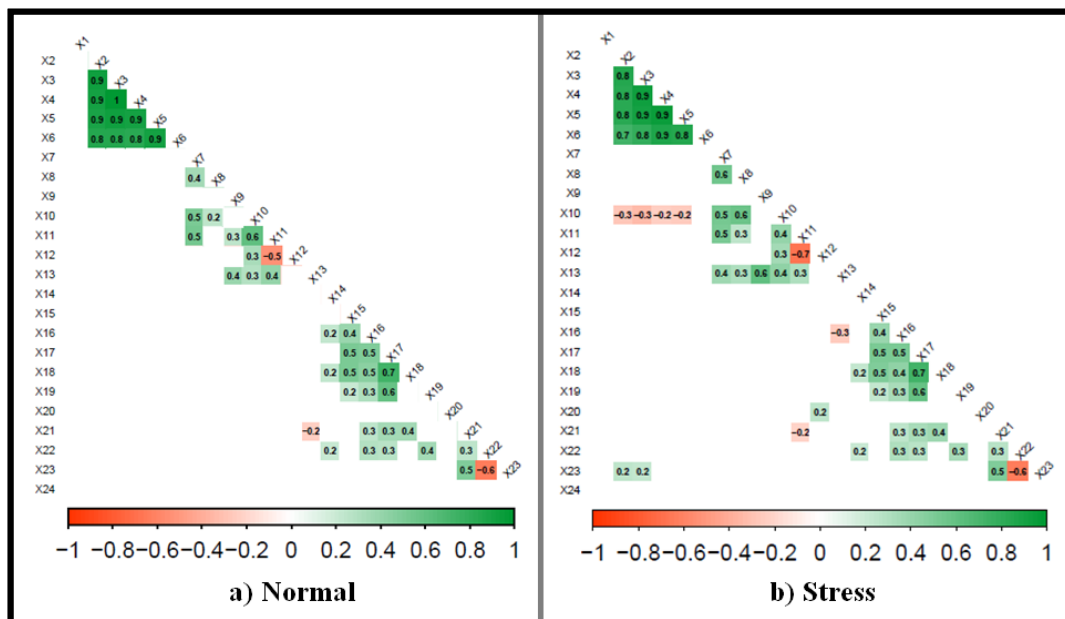
شکل ۱. ضرایب همبستگی پیرسون بین صفات مورد مطالعه در ژنوتیپ‌های ذرت تحت شرایط بدون تنش (a) و تنش کادمیوم (b). در نقشه هیتمپ (حرارتی)، جعبه‌های سبز و قرمز به ترتیب نشان‌دهنده ضرایب همبستگی مثبت و منفی هستند و افزایش شدت رنگ دلالت بر ضرایب بزرگ‌تر دارد. علاوه بر این، جعبه‌های سفید نشان‌دهنده ضرایب همبستگی غیرمعنی‌دار هستند.
