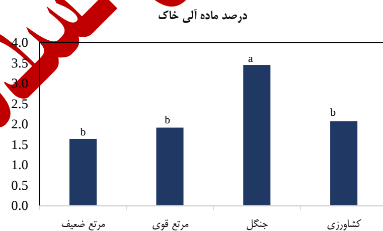
شکل ۴- تغییرات ماده آلی (درصد)، قابلیت هدایت الکتریکی (دسی‌زیمنس بر متر) و په‌اش در خاک کاربری‌های مختلف مورد مطالعه (میانگین‌های دارای حروف یکسان، از نظر آماری با استفاده از آزمون چند دامنه دانکن، در سطح احتمال ۵ درصد با یکدیگر اختلاف معنی‌دار ندارند).
