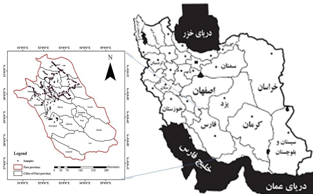
شکل ۱- منطقه مورد مطالعه به همراه موقعیت نقاط نمونه برداری شده در نیمه شمالی استان فارس
