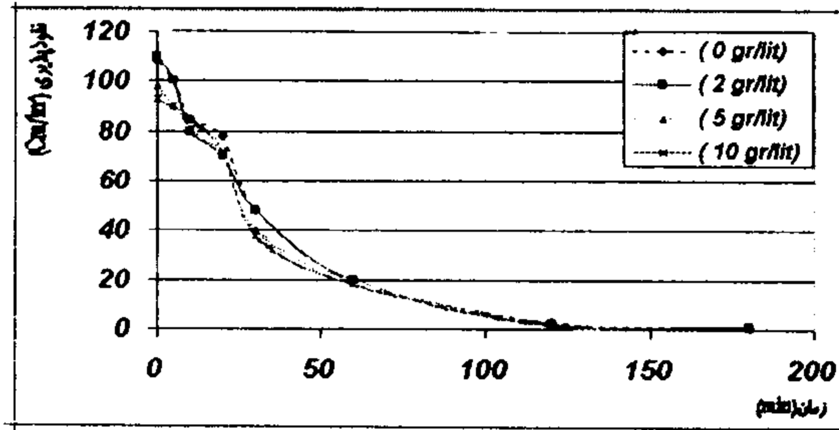
شکل ۸: منحنی‌های نفوذ در آزمایش مرحله پنجم (حوضچه b).
