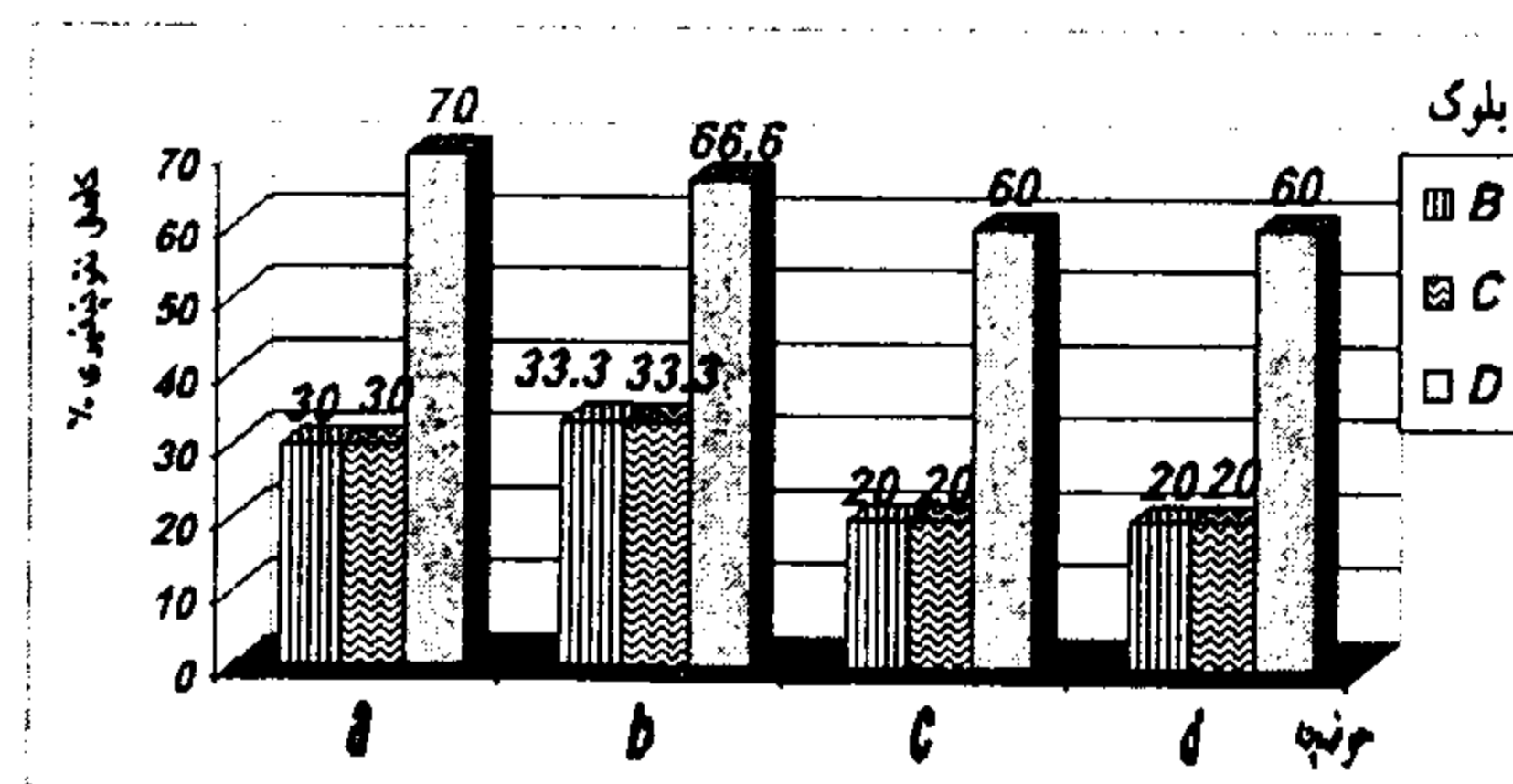
شکل ۳: میزان کاهش نفوذپذیری در آزمایشات مرحله سوم.
