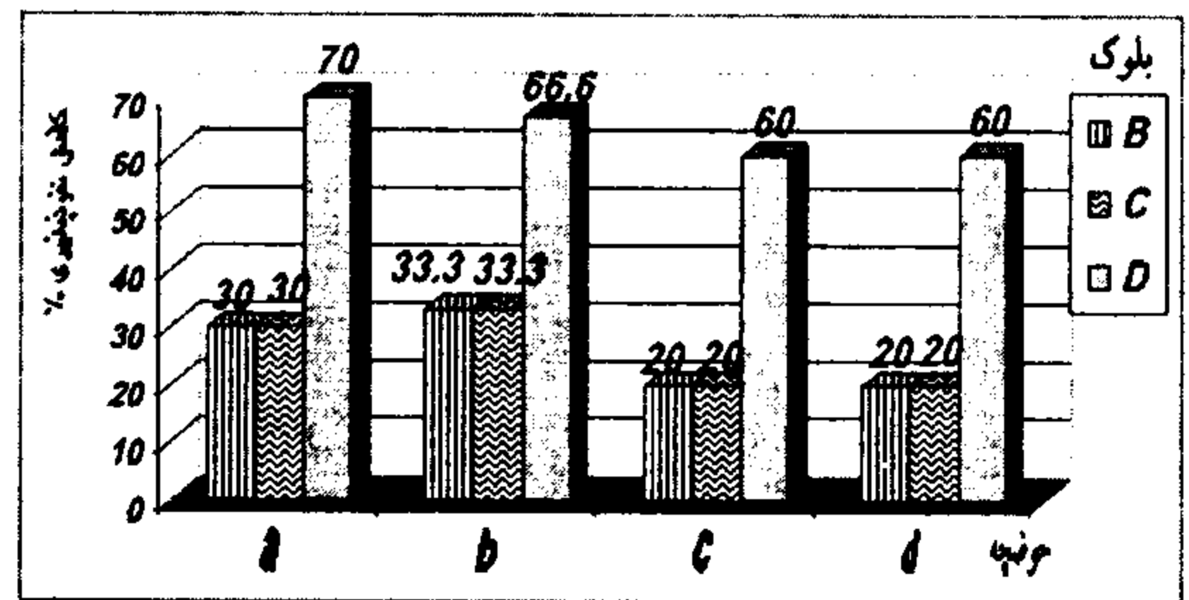
شکل ۴: میزان کاهش نفوذپذیری در آزمایشات مرحله چهارم.
