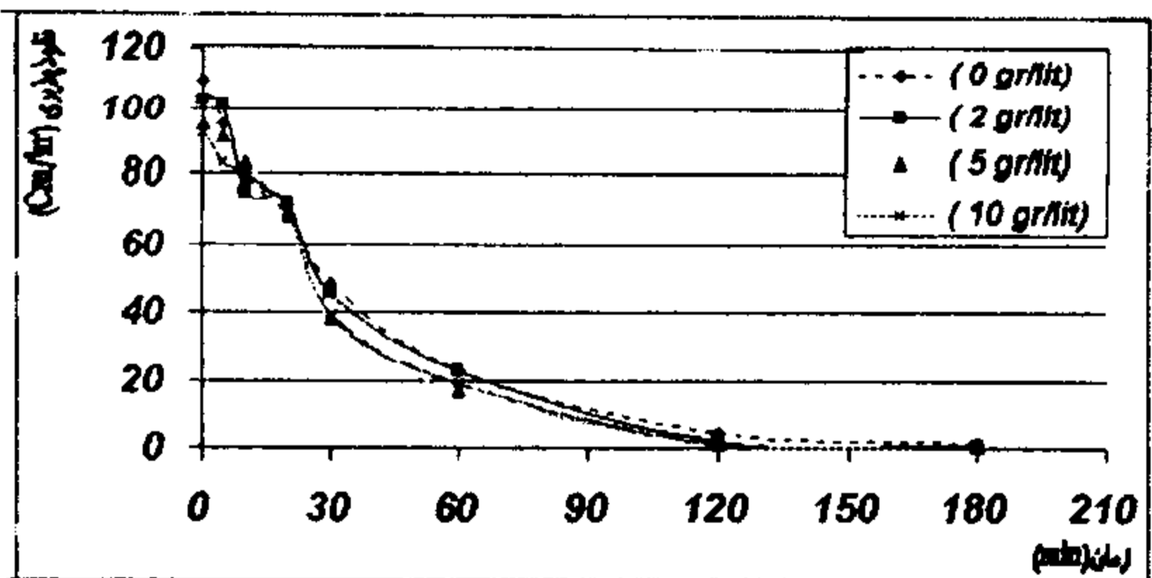
شکل ۱۰: منحنی‌های نفوذ در آزمایش مرحله پنجم (حوضچه d).
