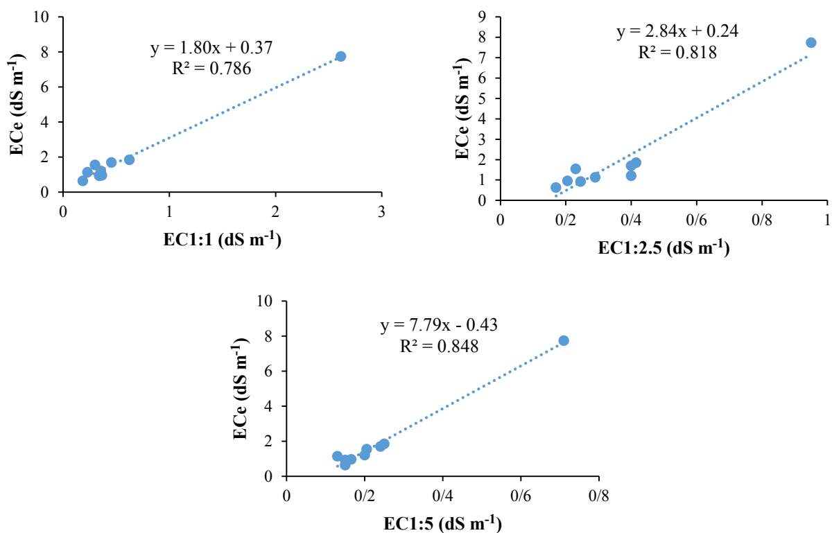
شکل ۴. رابطه بین قابلیت هدایت الکتریکی عصاره گل اشباع ( EC_e ) و نسبت‌های مختلف خاک به آب ( EC_{1:1} ، EC_{1:2.5} و EC_{1:5} ) در خاک‌های درشت بافت ( n=9 )
