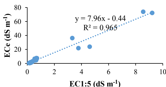
شکل ۲. رابطه بین قابلیت هدایت الکتریکی عصاره گل اشباع ( EC_e ) و نسبت‌های مختلف خاک به آب ( EC_{1:1} ، EC_{1:2.5} و EC_{1:5} ) در خاک‌های ریز بافت ( n=33 )
