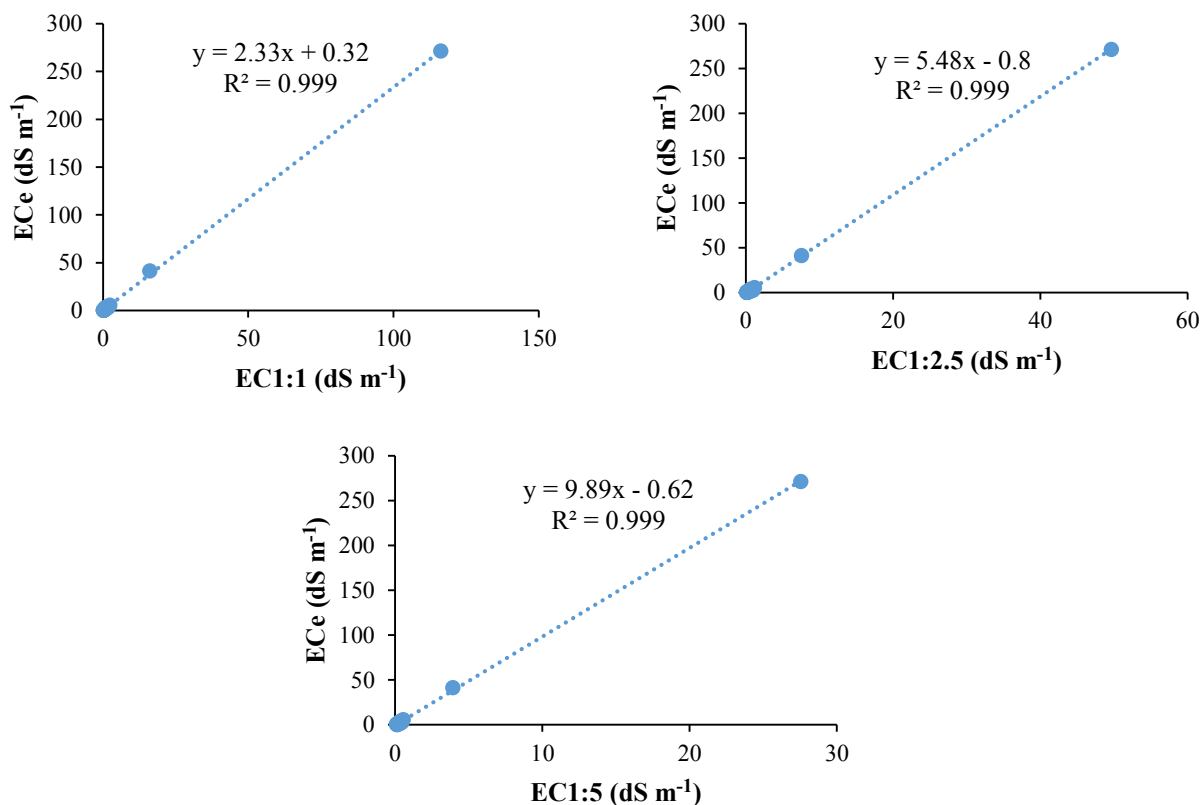
شکل ۳. رابطه بین قابلیت هدایت الکتریکی عصاره گل اشباع ( EC_e ) و نسبت‌های مختلف خاک به آب ( EC_{1:1} ، EC_{1:2.5} و EC_{1:5} ) در خاک‌های متوسط بافت ( n=22 )
