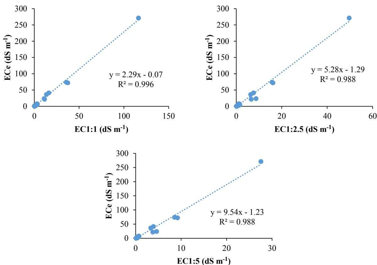
شکل ۵. روابط توسعه داده بین قابلیت هدایت الکتریکی عصاره گل اشباع ( EC_e ) و نسبت‌های مختلف خاک به آب ( EC_{1:1} ، EC_{1:2.5} و EC_{1:5} ) با استفاده از کل داده‌ها ( n=64 )
