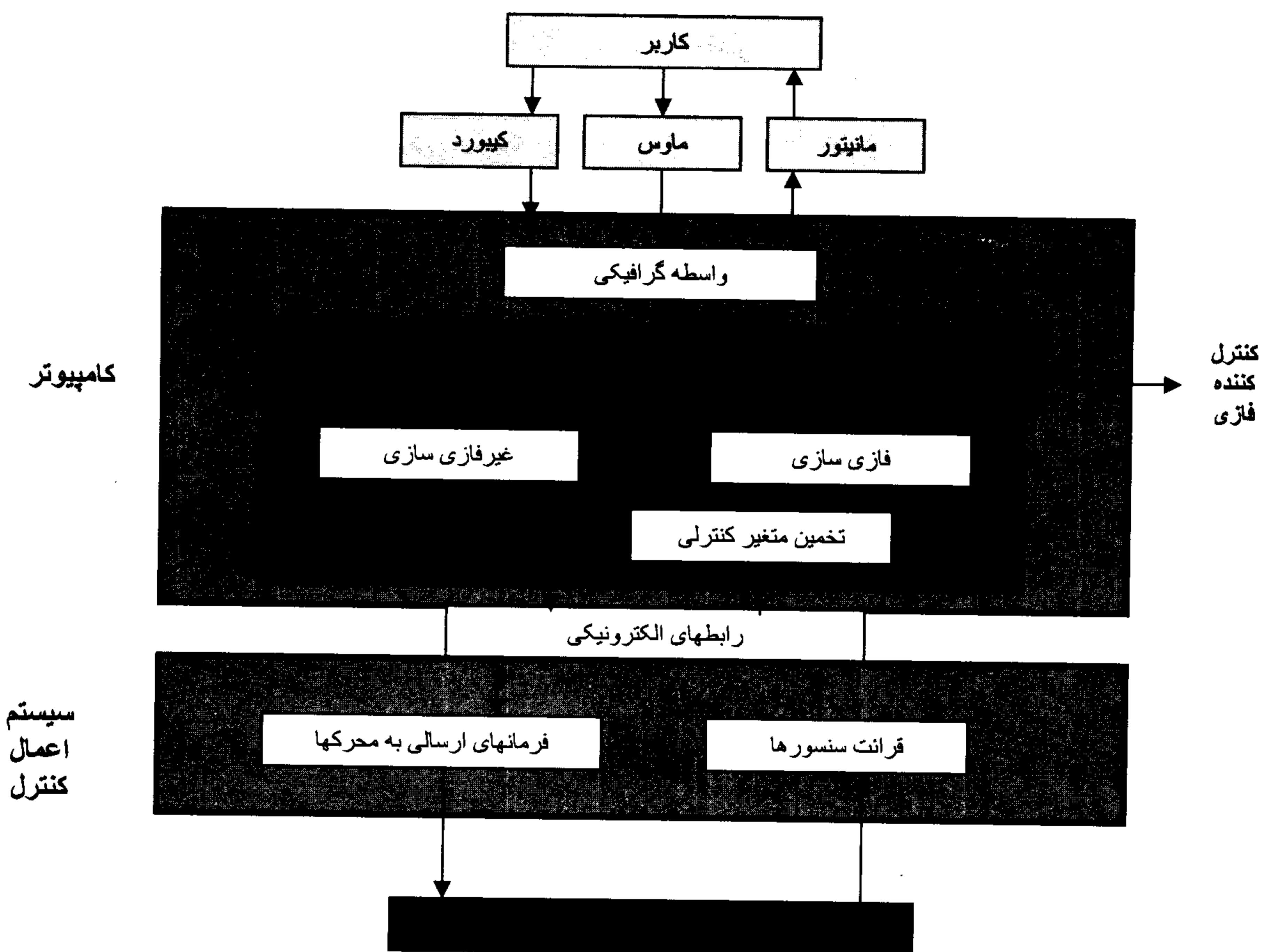
شکل ۱۳: معماری سیستم کنترل سلول فلوتاسیون ستونی.
