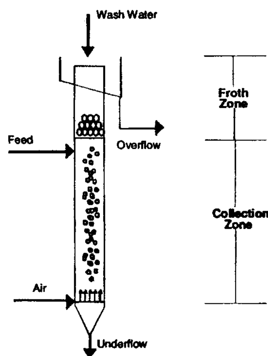
شکل ۱: نمایی کلی از یک سلول فلوتاسیون ستونی [۱].
