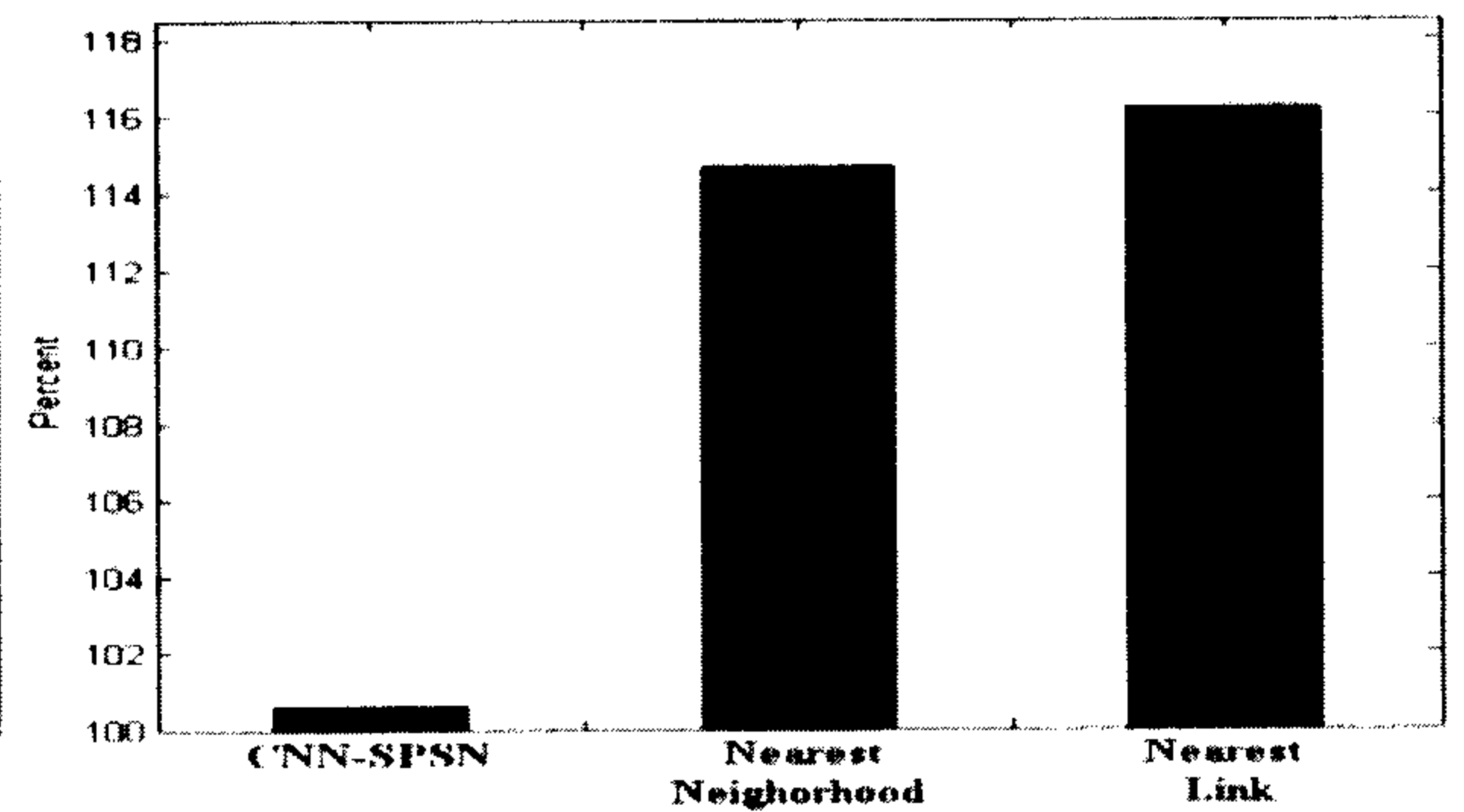
شکل ۸: طول متوسط مسیرهای ۵۰ شهری پیشنهاد شده توسط الگوریتم‌های CNN-SPSN (ستون اول)، نزدیکترین همسایه (ستون دوم) و نزدیکترین کمان (ستون سوم) نسبت به طول مسیر کوتاه‌تر برای ۲۰۰ توزیع ۱۰۰ شهری.
