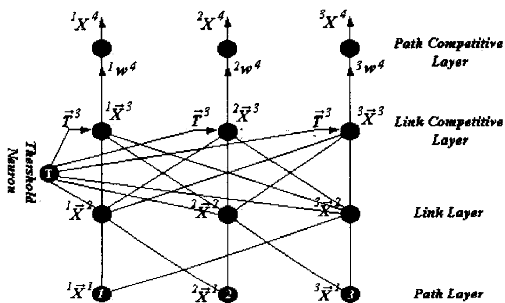
شکل ۲: شبکه عصبی پیشنهادی اولیه.
