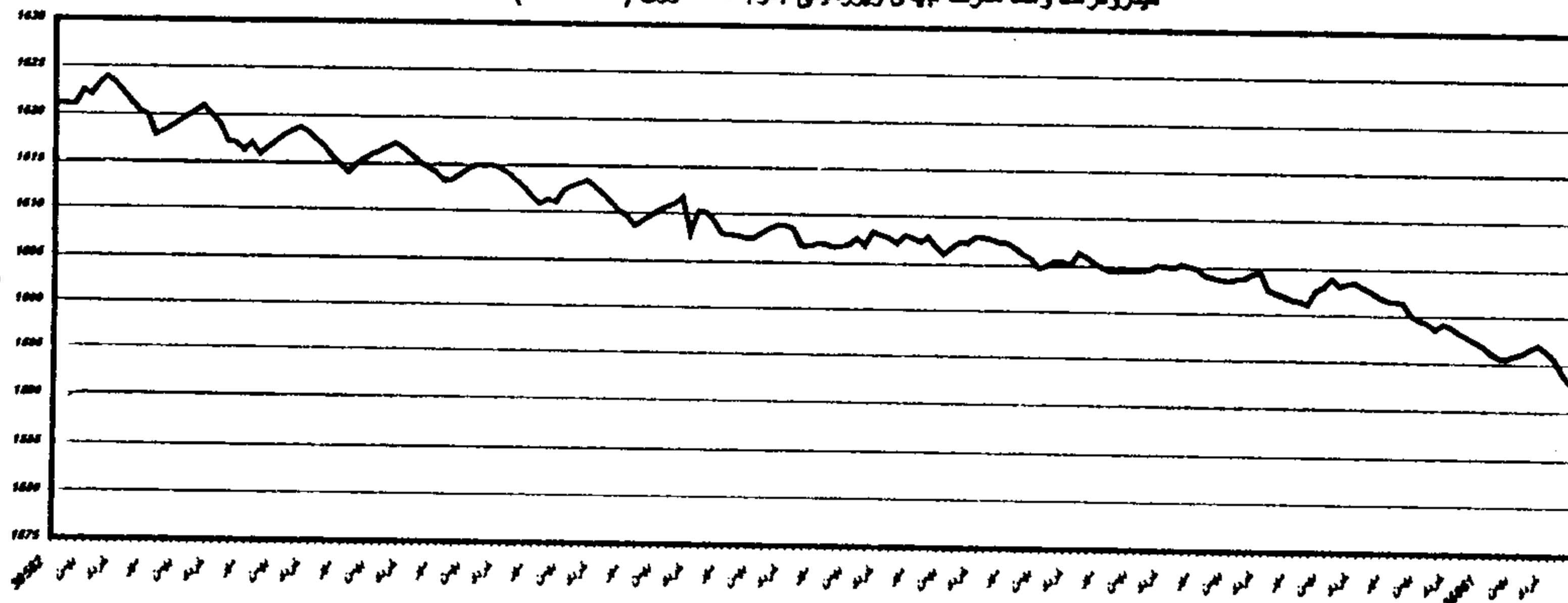
هیدروگراف واحد آبهای زیرزمینی دشت کبودرآهنگ (۱۳۶۱-۷۸)
