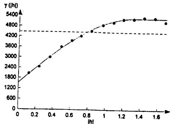
شکل ۳- واریوگرام همه جانبه هدایت الکتریکی عناصره اشباع که در آن h بر حسب کیلومتر و \gamma(h) بر حسب (\text{ds/m})^2 می باشد
