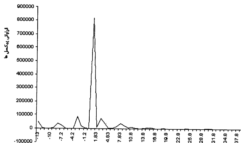
شکل ۲- فراوانی پیکسل‌ها در برابر مقادیر Y در پهنه بندی خطر زمین لغزش به روش رگرسیون چند متغیره (MR)
