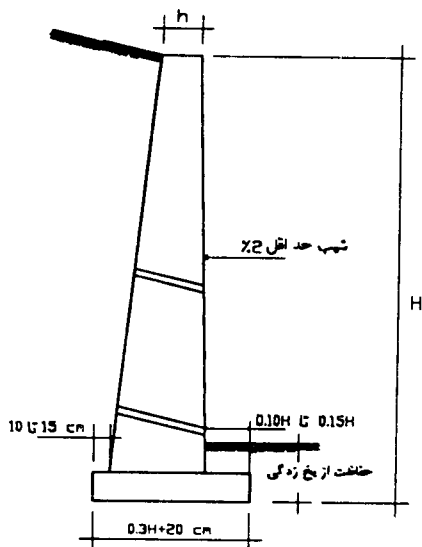
شکل ۳. ابعاد تقریبی قابل استفاده برای دیوارهای نگهبان وزنی.
