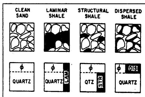
شکل ۳: اشکال مختلف توزیع شیل و تاثیر آن بر تخلخل سازند.
