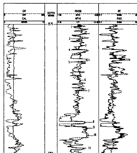
شکل ۸: نمودارهای درون چاهی و نقاط انتخاب شده در یک چاه دیگر.
