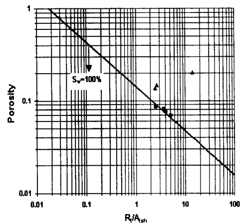
شکل ۵: نمودار متقاطع بیکت رسم شده بر اساس داده های مندرج در جدول (۱).
