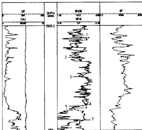
شکل ۴: نمودارهای درون چاهی و نقاط انتخاب شده در یکی از چاهها.
