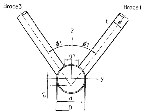
ب - مقطع عرضی اتصال KK در صفحه Y-Z
