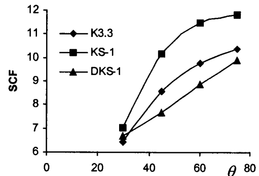
شکل ۱۵: تغییرات SCF بر حسب \theta .
