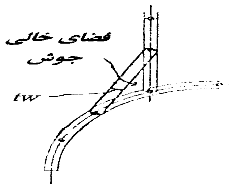
شکل ۴: جوش مورد استفاده.
