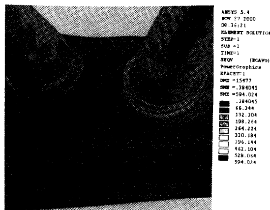
شکل ۱۰: نتیجه تحلیل اتصال DKS-1.
