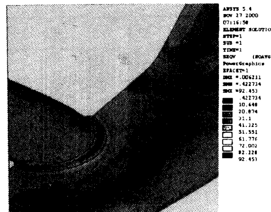
شکل ۷: نتیجه تحلیل اتصال K3.3.
