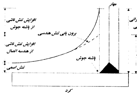
شکل ۲: تشنش بحرانی هندسی و موضعی.
