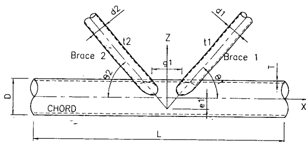
ج - مقطع طولی اتصال KK در صفحه X-Z
