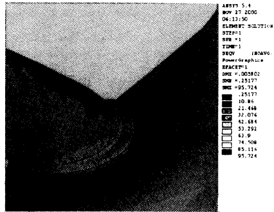
شکل ۶: نتیجه تحلیل اتصال K3.1.
