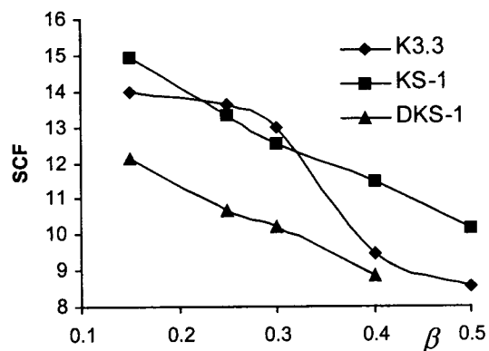
شکل ۱۲: تغییرات SCF بر حسب β.
