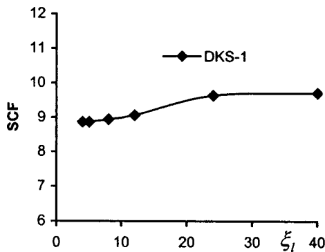
شکل ۱۷: تغییرات SCF بر حسب \xi_1 .
