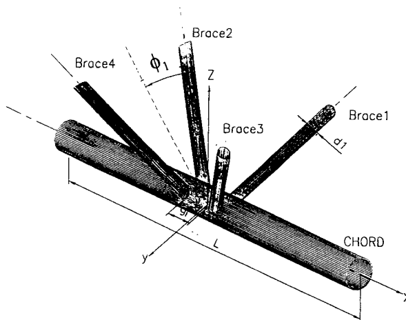
الف - اتصال KK در دستگاه مختصات سه بعدی
