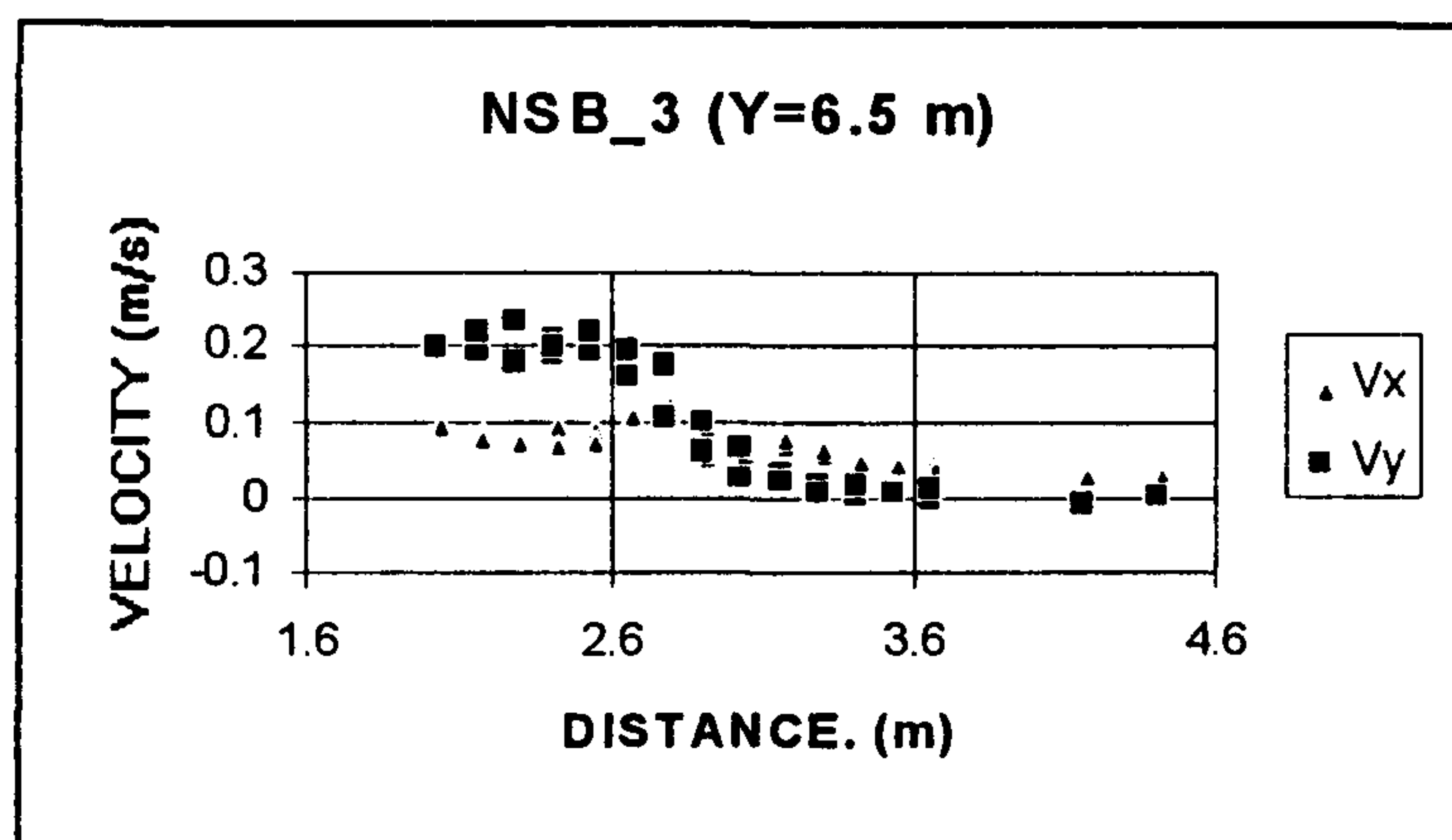
شکل ۶: مثالی از توزیع سرعت جریان ناشی از امواج؛ V_y سرعت جریان موازی ساحل و V_x سرعت جریان عمود بر ساحل میباشد.
