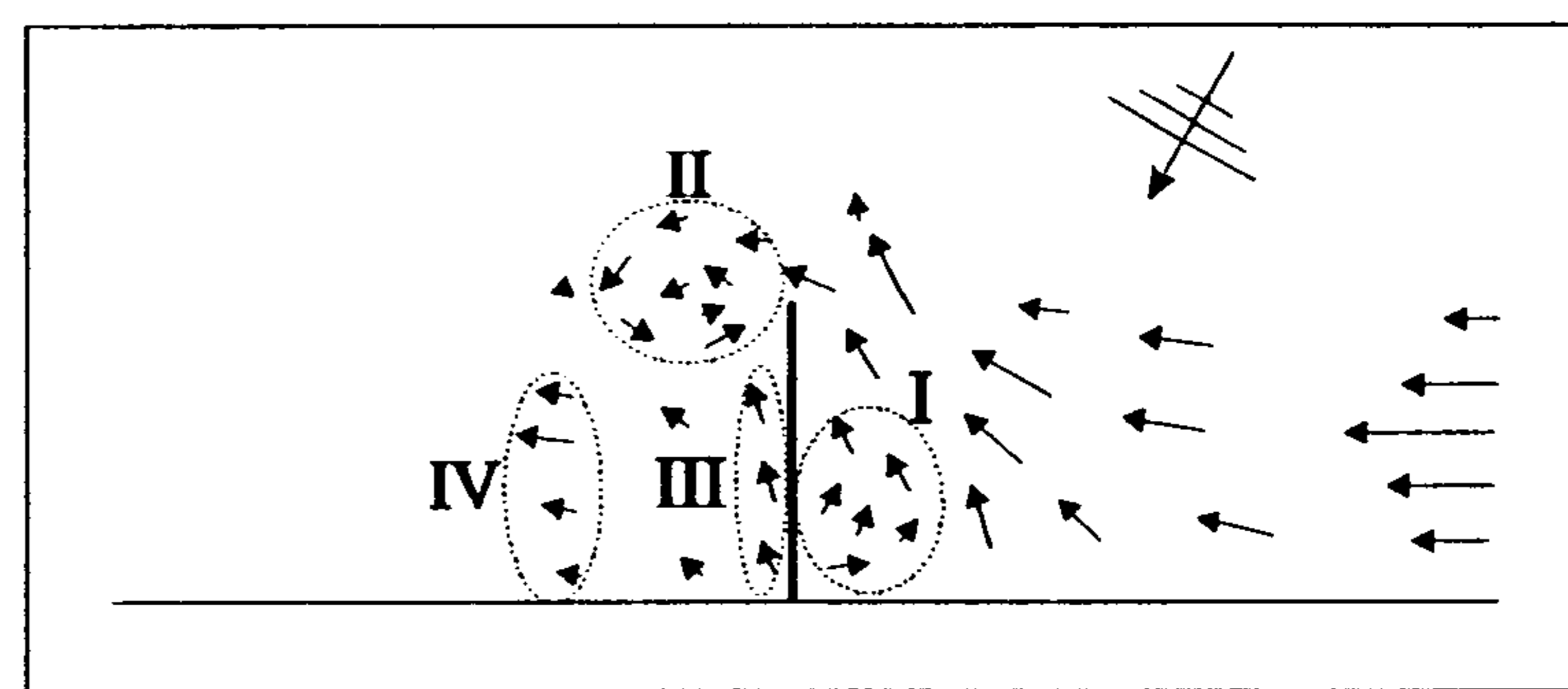
شکل ۲۳: الگوی عمومی جریانات نزدیک ساحل در اطراف یک آبشکن.
