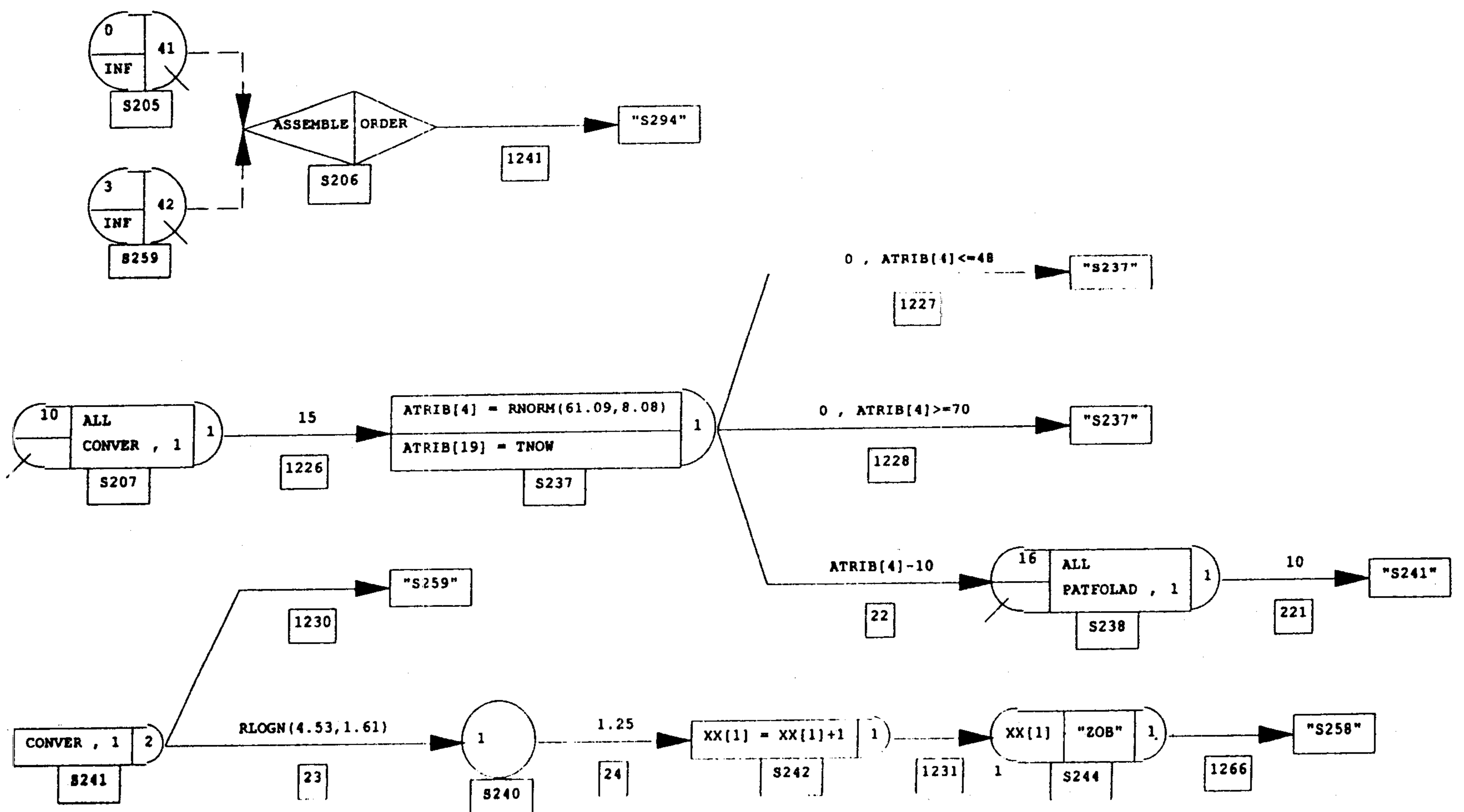
نمودار ۳: بخشی از شبکه Awesim آماده کردن ذوب (Z3).
