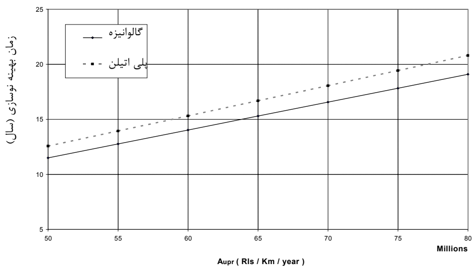
شکل ۸: مقایسه آنالیز حساسیت زمان نوسازی لوله های پلی اتیلن و گالوانیزه نسبت به پارامتر A_{uپر} .
