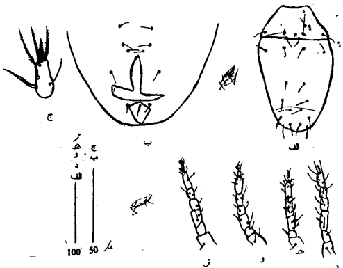
شکل ۲۷- کنه ماده Metapronematus sp. (Original)
