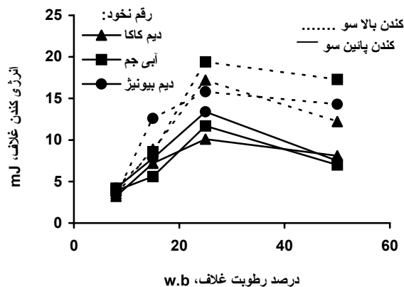
شکل ۱۱- مقایسه تاثیر رطوبت بر انرژی مصرفی برای کندن غلاف ارقام مختلف در سرعت ۵۰۰ میلیمتر بر دقیقه.
