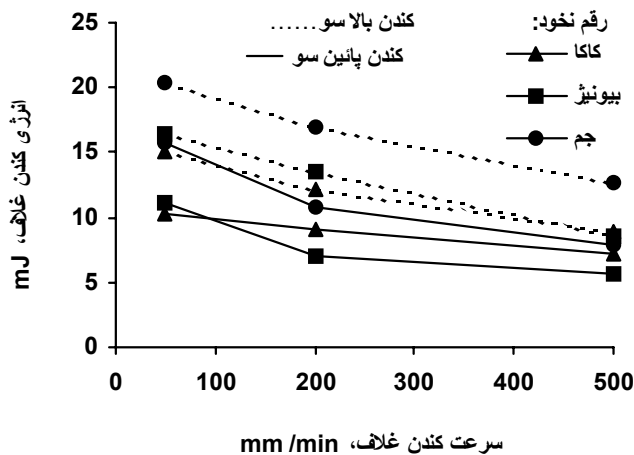
شکل ۱۲- مقایسه تاثیر سرعت کندن بر انرژی مصرفی برای کندن غلاف ارقام مختلف در رطوبت ۱۵٪.
