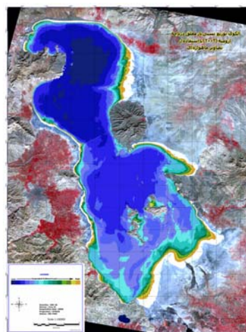
۹ د: پراکندگی مواد معلق آب دریاچه ارومیه در سال ۲۰۰۲
