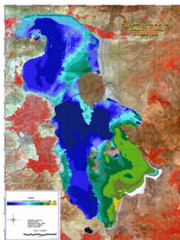
۹ ج: پراکندگی مواد معلق آب دریاچه ارومیه در سال ۲۰۰۱
