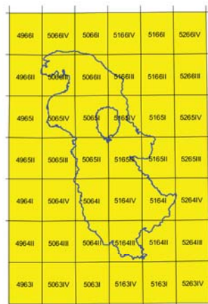
شکل ۴ موزائیک نقشه های توپوگرافی دریاچه ارومیه
