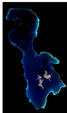
محدوده آب دریاچه ۲۰۰۲
