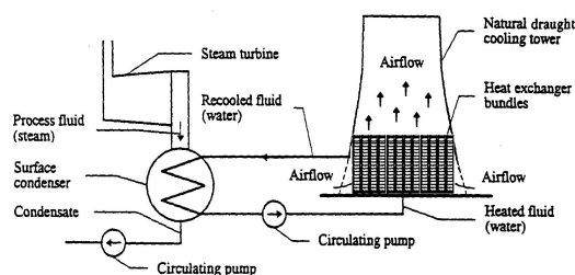
شکل ۱: چرخه قدرت با برج خنک کن هلر.
