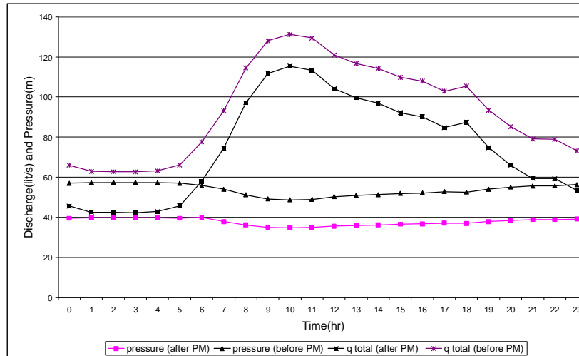
شکل ۶: نمودار فشار و دبی کل شبکه در هر ساعت قبل و بعد از تعدیل فشار (PM).
