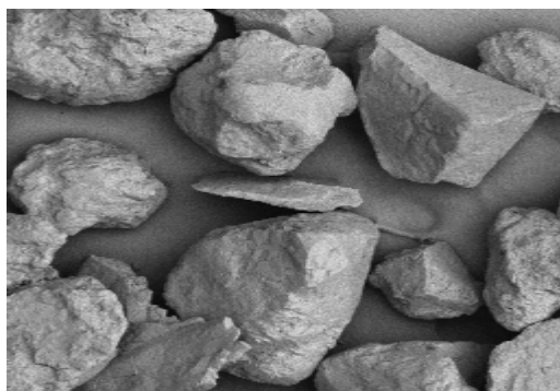
شکل ۳: تصویر میکروسکوپی دانه‌های ماسه فیروزکوه [۸].
