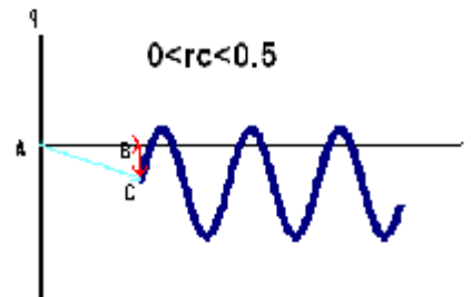
شکل ۵-الف: آزمایش با برگشت تنش‌ها به سمت کششی.
