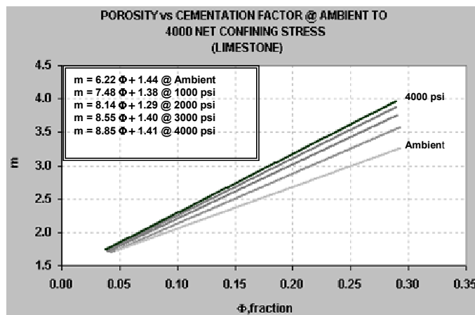
شکل ۱۸: نمودار ضریب سیمان‌شدگی بر حسب تخلخل برای نمونه‌های گرینستون برای فشار همه‌جانبه موثر از شرایط فشار محیط تا ۴۰۰۰ پوند بر اینچ مربع.
