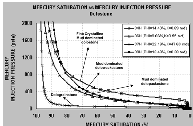
شکل ۱۵: نمودار فشار موئینگی جیوه در دولوستون.
