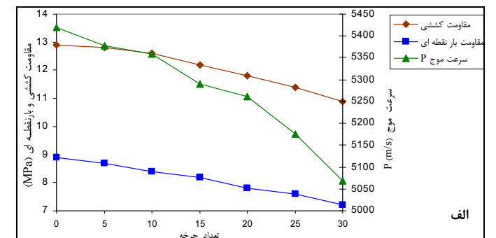
شکل ۱۰- تغییرات ویژگی‌های مهندسی نمونه‌ها با افزایش تعداد چرخه های انجماد و ذوب آب الف- ایگنریت نائین ب- داسپت بزد.
