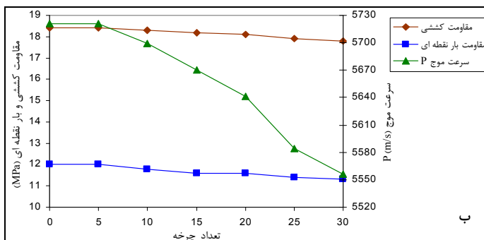
شکل ۱۰- تغییرات ویژگی‌های مهندسی نمونه‌ها با افزایش تعداد چرخه های انجماد و ذوب آب الف- ایگنریت نائین ب- داسپت بزد.
