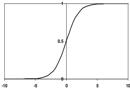
شکل ۲- تابع سیگموئید
