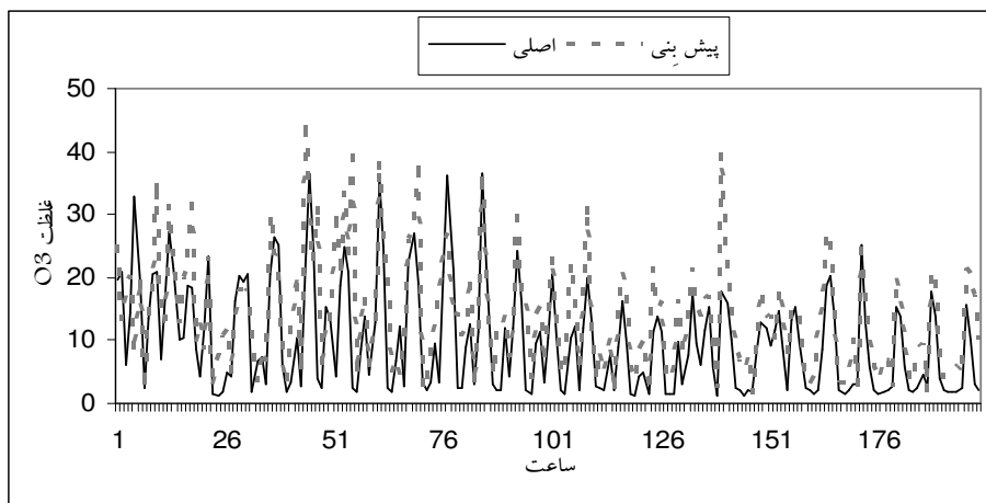
شکل ۶- همبستگی بین داده‌های اصلی و پیش بینی برای غلظت ازن به صورت ساعتی در شهر تبریز، با مدل خطی (MLR)
