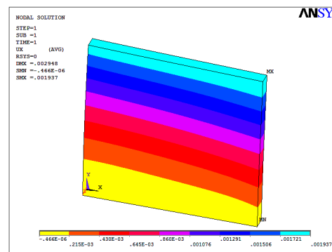
شکل 17: توزیع تغییرشکل جانبی دیوار در دو حالت دقیق و همگن شده.
