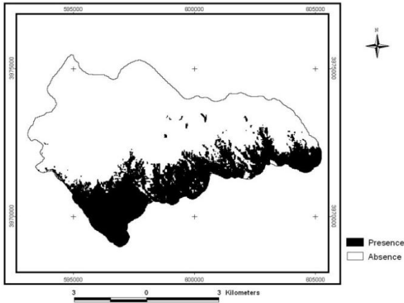
شکل ۸. نقشه‌ی پیش‌بینی حضور گونه‌ی Astragalus sieversianus
