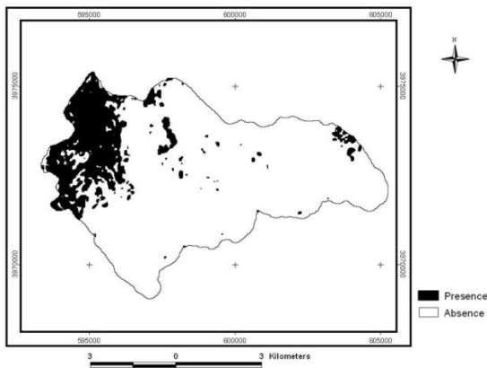
شکل ۱۰. نقشه‌ی پیش‌بینی گونه‌ی Astragalus microcephalus
