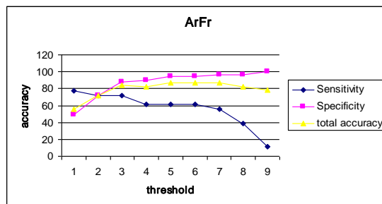
شکل ۱۳. نمودار حساسیت، خصوصیت و صحت کلی در احتمالات مختلف
