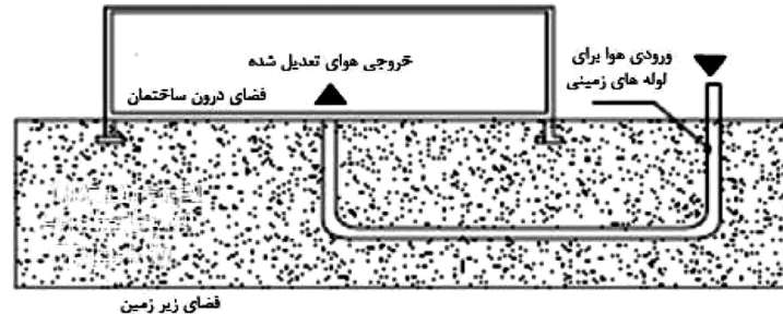
تصویر ۲- نمودار عملکرد سیستم لوله های زمینی به صورت شماتیک.
