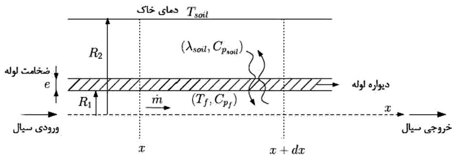
تصویر ۶- نمودار تبادل حرارتی بین هوای درون لوله و خاک به صورت شماتیک. ماخذ: (Derbel et al., 2010)
