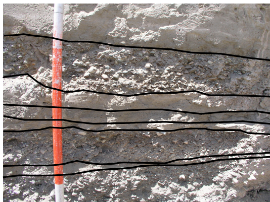
شکل ۱۱: مقطع قسمتی از رودخانه جاجرود که لایه‌های متفاوت آبرفتی حاصل جریان‌های متفاوت را نشان می‌دهند (لایه‌های سیلت و رس به همراه لایه‌های نازکی از ماسه و لایه‌های ضخیم با آبرفت‌های درهم ناهمگن)
