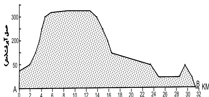
شکل ۳ عمق آبرفت در امتداد محور طولی مخروط افکنه (با استفاده از نقشه Ananyos، ۱۹۶۴)
