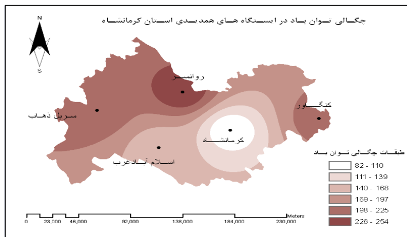
شکل ۷. نقشه‌ی پتانسیل انرژی باد سالانه‌ی استان کرمانشاه
