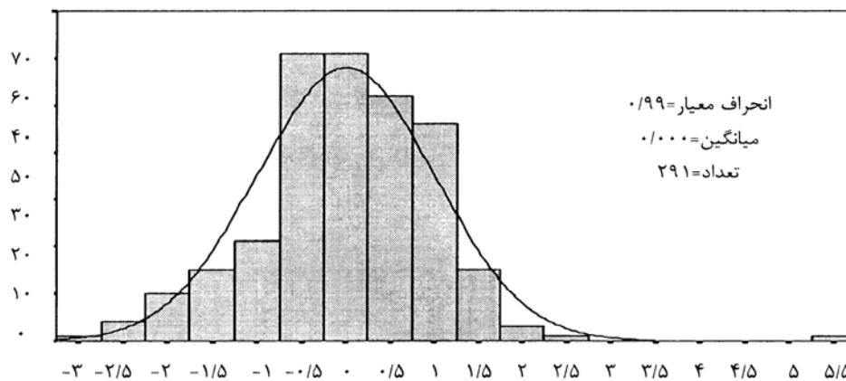
شکل ۱ - نمودار هیستوگرام
