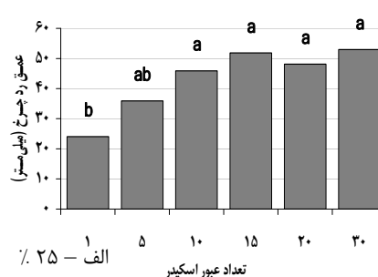
شکل ۵- مقایسه میانگین افزایش عمق شیاری در اثر تعداد ترددهای مختلف اسکیدر در سه گروه رطوبتی خاک؛ رطوبت ۲۵ درصد (الف)، ۳۵ درصد (ب) و ۴۵ درصد (ج). حروف لاتین نامتشابه نشانگر معنی‌دار بودن اختلاف میانگین‌ها در سطح احتمال ۹۵ درصد است
