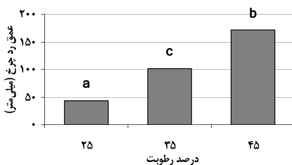
شکل ۴- اثر مستقل درصد رطوبت خاک بر روی عمق شیاری در خاک‌های مسیر چوب‌کشی. حروف لاتین نامتشابه نشانگر معنی‌دار بودن اختلاف میانگین‌ها در سطح احتمال ۹۵ درصد است
