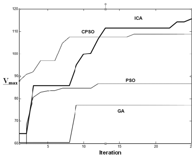
نمودار ۵. مقایسه منحنی‌های همگرایی الگوریتم‌های ICA، GA، PSO و CPSO برای مسئله یکسان
