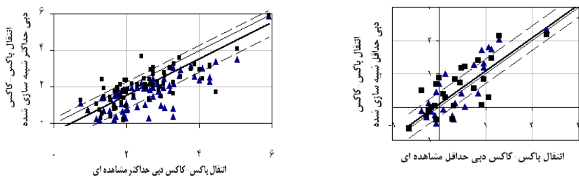
شکل ۳. نمودار پراکنش انتقال باکس-کاکس دبی‌های حداقل مشاهده‌ای و شبیه‌سازی‌شده (سمت راست) و دبی‌های حداکثر مشاهده‌ای و شبیه‌سازی‌شده (سمت چپ) با استفاده از مدل تانک (▲) و SIMHYD (■). در شکل خطوط نقطه‌چین نیم‌ساز، خطوط ممتد کم‌رنگ انحراف معیار، و خطوط ممتد پُررنگ نشان‌دهنده انحراف میانگین است.
