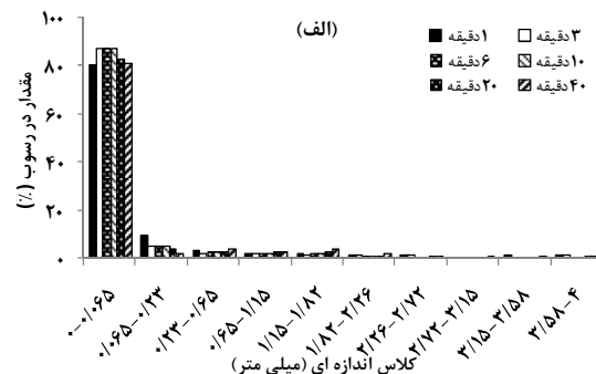
شکل ۴. تغییرات توزیع اندازه ذرات رسوب در نمونه خاک گیلوان در قدرت جریان‌های الف (۰.۱۲، ب) ۰.۲، ج) ۰.۳، د) ۰.۴، ه) ۰.۶، و) ۰.۸ وات بر متر مربع
