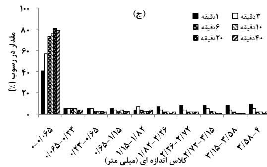
شکل ۵. تغییرات توزیع اندازه ذرات رسوب با زمان در نمونه خاک جنگلی در قدرت جریان‌های الف (۰.۳، ب) ۰.۴، ج) ۰.۶، د) ۰.۸ وات بر متر مربع
