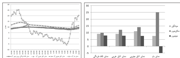
تصویر ۷- نمودار تغییرات دمای اتاق های مورد بررسی خانه امینیان (سمت چپ)، نمودار میانگین دمای بیشینه و کمینه اتاق های مورد بررسی (سمت راست). ۱۳۸۹/۹/۱۹
