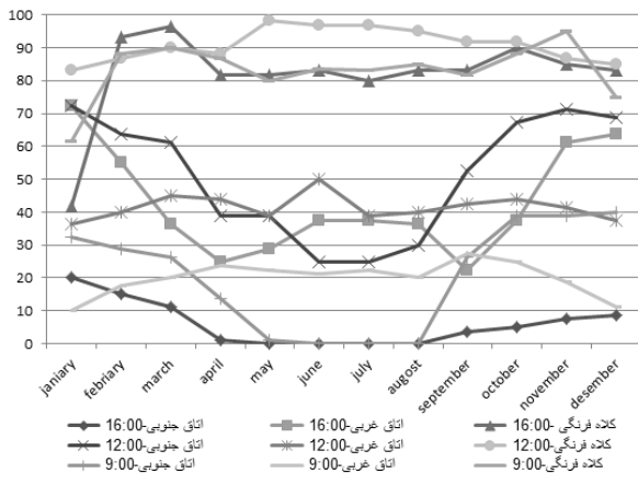
تصویر ۱۱- نمودار درصد مساحت اتاق دارای میزان روشنایی ۳۰۰-۹۰۰ لوکس برای زمان های صبح و ظهر و عصر.
