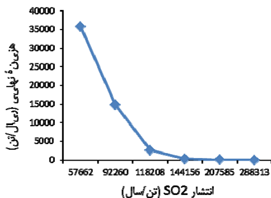
شکل ۲. منحنی هزینه کاهش آلودگی برای کنترل SO 2 مجتمع مس سرچشمه
