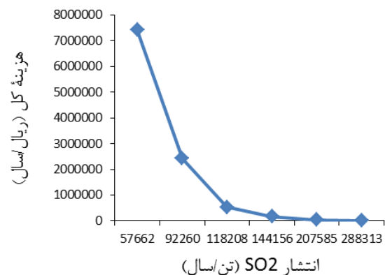
شکل ۳. منحنی هزینه کاهش آلودگی برای کنترل SO 2 مجتمع مس سرچشمه
