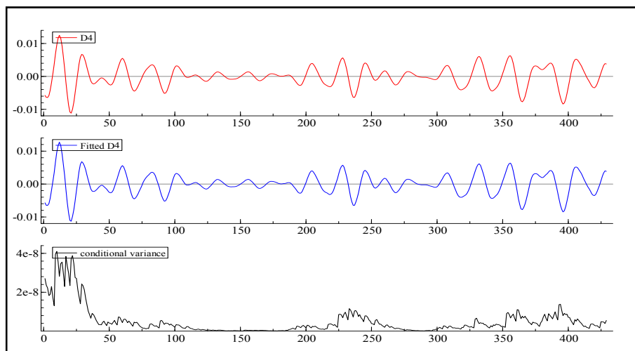
شکل ۶. مقیاس D_\epsilon(t) موجک و تخمین مدل ARMA-EGARCH
