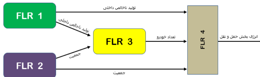
شکل ۱. ساختار مدل رگرسیون خطی فازی طراحی شده
