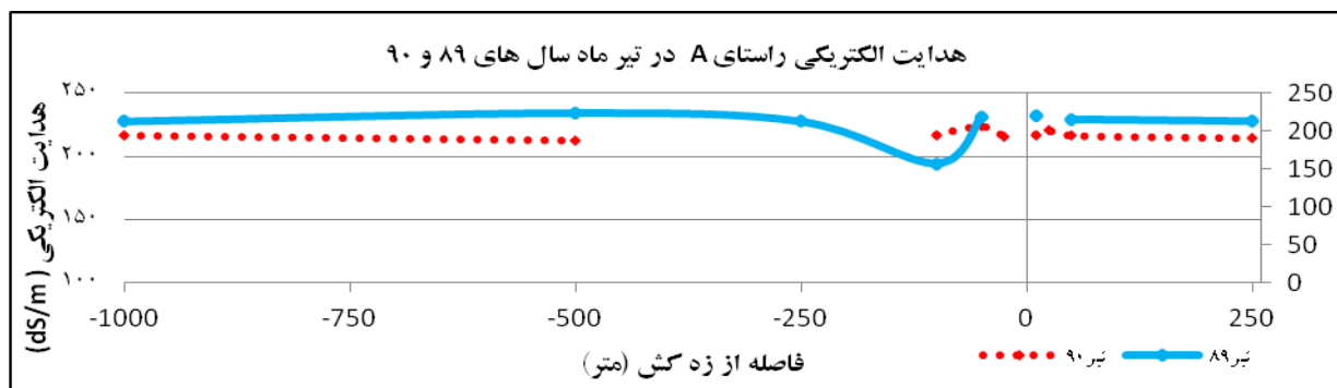
شکل ۷. تغییرات شوری آب زیر سطحی در فاصله زمانی تیر ۱۳۸۹ تا تیر ۱۳۹۰ در چاهک‌های راستای A
