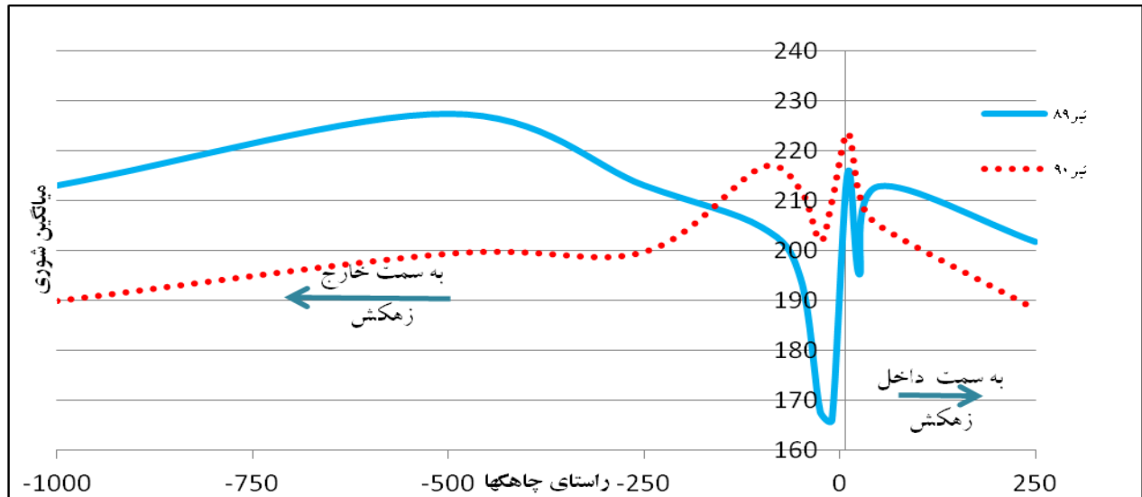
شکل ۶. میانگین تغییرات شوری آب زیر سطحی در فاصله زمانی تیر ۱۳۸۹ تا تیر ۱۳۹۰ در همه چاهک‌ها
