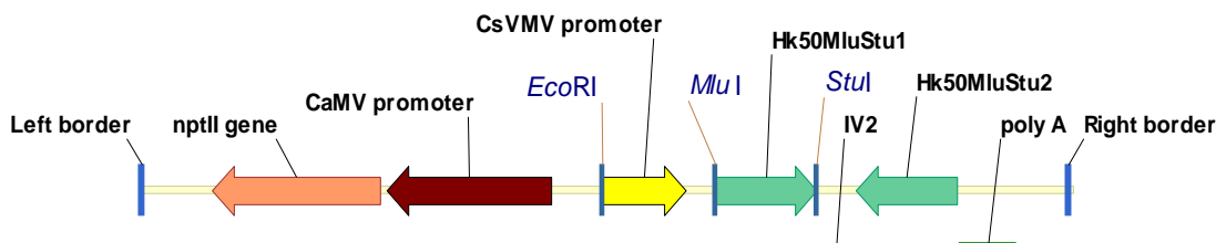
شکل ۱. نقشه سازه سنجاق سری در حد فاصل نواحی مرزی RB و LB به طول ۴۴۲۳ باز
