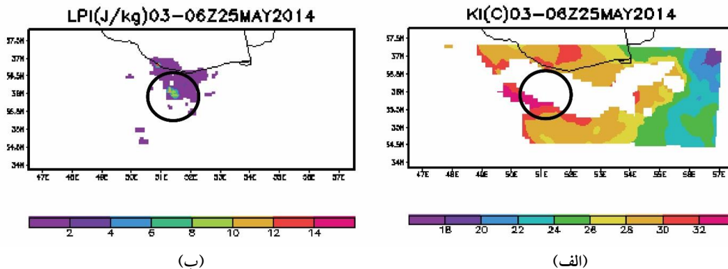
شکل ۵. میانگین سه ساعته شاخص KI (الف) و LPI (ب) برای ساعت ۰۳:۰۰ تا ۰۶:۰۰ گرینویچ ۲۵ می ۲۰۱۴ در منطقه ایران
