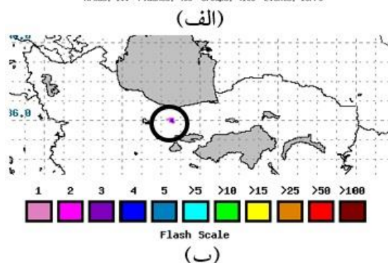
شکل ۴. درخش‌های آذرخش حاصل از سنجنده LIS برای ۹ دسامبر ۲۰۱۳
