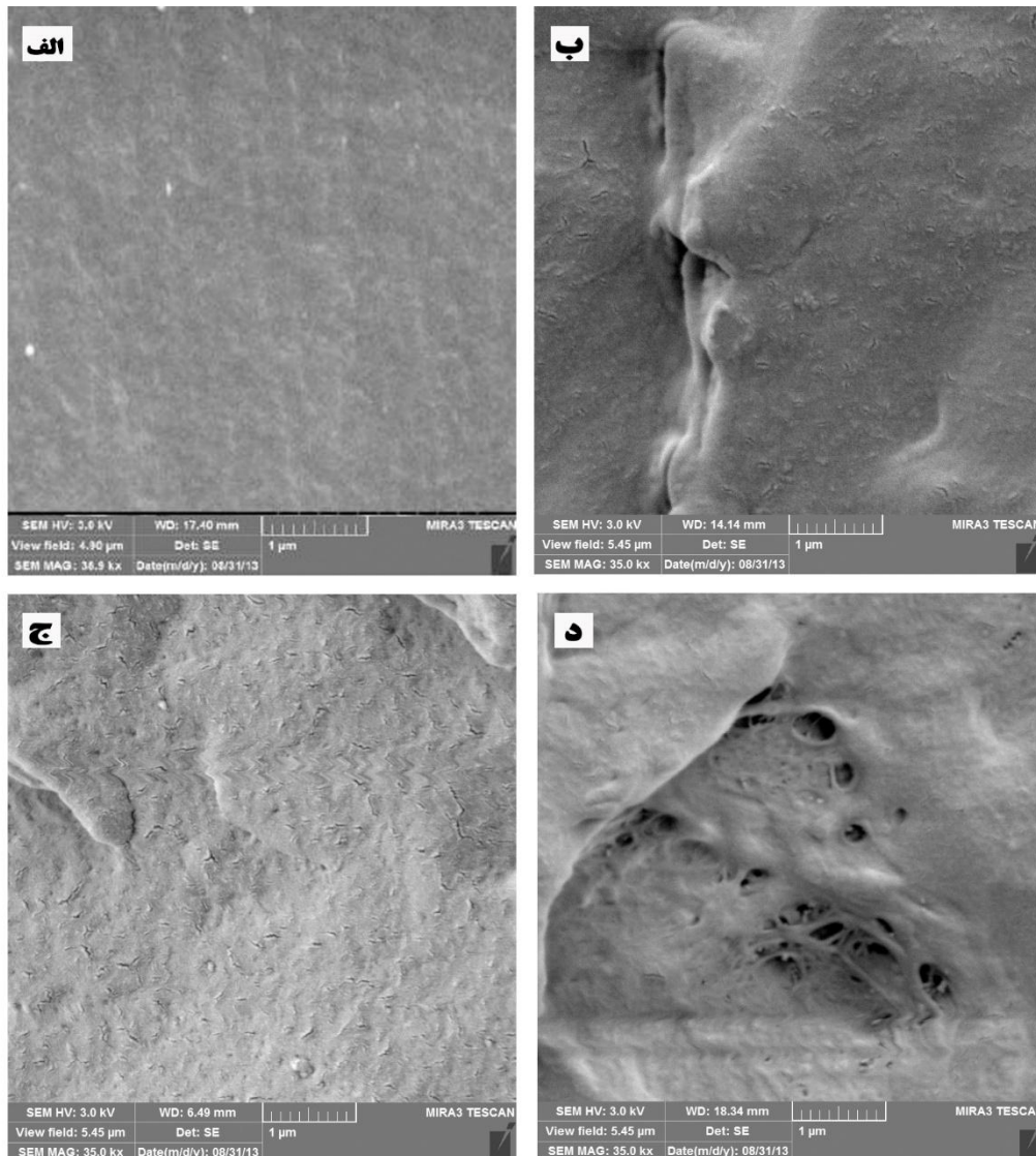
شکل ۱. تصاویر میکروسکوپ الکترونی روبشی مورفولوژی سطح شکست: (الف) پلی اتیلن سبک خالص، (ب) نانوکامپوزیت حاوی ۵/۰ درصد نانوقره، (ج) نانوکامپوزیت حاوی ۵/۰ درصد نانواکسید روی، و (د) نانوکامپوزیت حاوی ۵/۰ درصد نانواکسید مس
