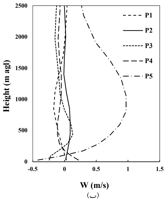
شکل ۷. همانند شکل ۵، برای کمیت سرعت قائم.
