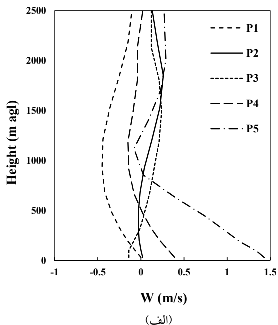
شکل ۷. همانند شکل ۵، برای کمیت سرعت قائم.
