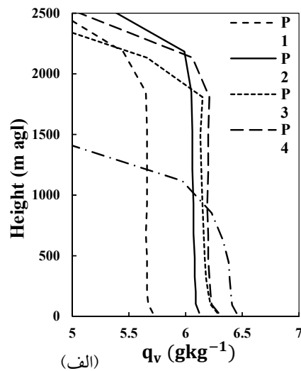
شکل ۶. همانند شکل ۵، برای کمیت نسبت آمیختگی بخار آب.
