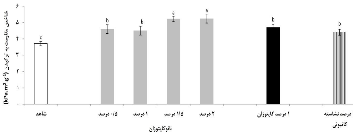
شکل ۵. تأثیر افزودن نانوکایتوزان، کایتوزان و نشاسته بر شاخص مقاومت به ترکیدن در کاغذهای بازیافتی (حروف لاتین گروه‌بندی دانکن در سطح ۱ درصد خطا نشان می‌دهند)
