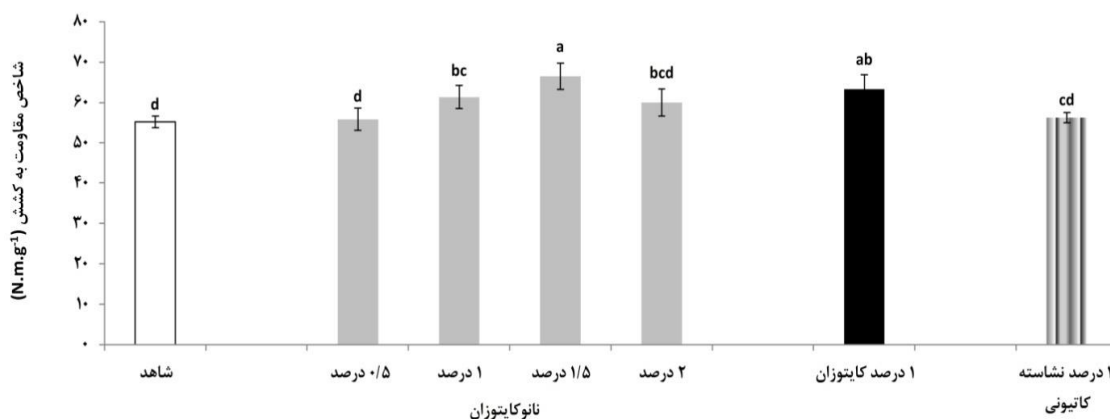
شکل ۴. تأثیر افزودن نانوکایتوزان، کایتوزان و نشاسته بر شاخص مقاومت به کشش در کاغذهای بازیافتی (حروف لاتین گروه‌بندی دانکن در سطح ۱ درصد خطا نشان می‌دهند)
