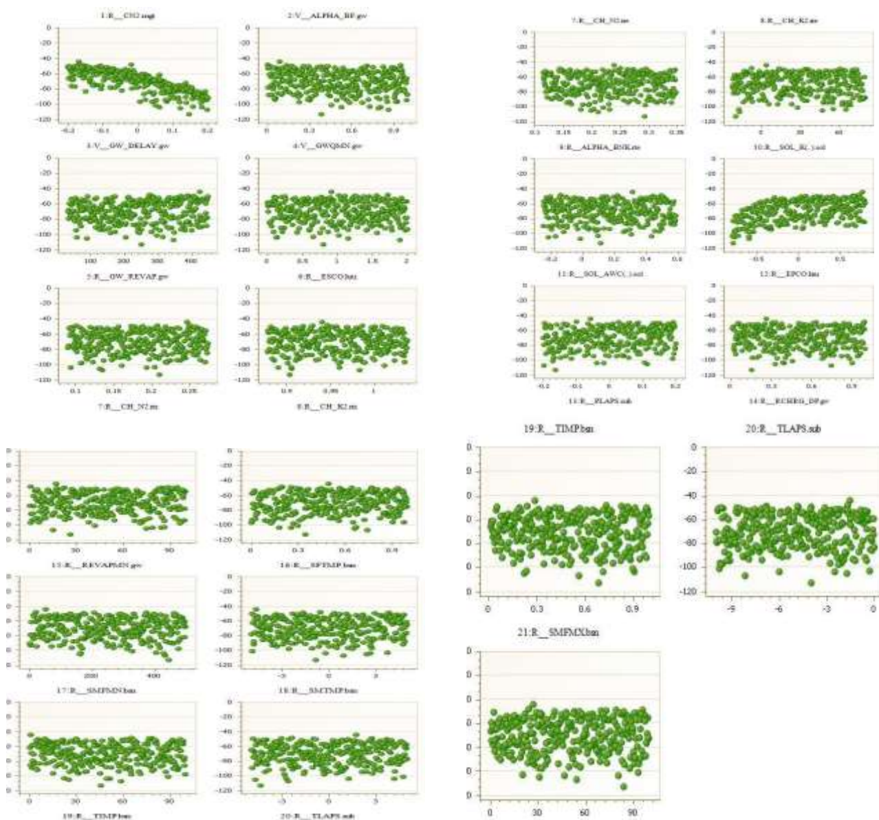
شکل ۵. ترسیم نقطه‌ای ۲۱ پارامتر با حساسیت بالا در مرحله کالیبراسیون با نرم‌افزار الحاقی SUFI2 مدل SWATCUP
