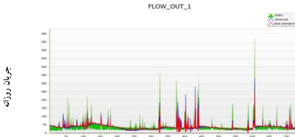
شکل ۶. نمودار جریان روزانه مشاهده‌شده و شبیه‌سازی‌شده از ۲۱ پارامتر با حساسیت بالا در مرحله اعتبارسنجی مدل SWATCUP با استفاده از نرم‌افزار الحاقی SUFI2
