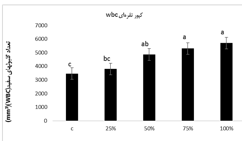
نمودار ۲- تغییرات میانگین (میانگین \pm SD) میزان گلبول‌های سفید خون ماهی کپور نقره‌ای در غلظت‌های مختلف پس‌آب ( P < 0.05 ). (حروف غیر مشابه اختلاف معنی‌دار را نشان می‌دهد).
