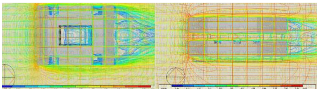
تصویر ۵- الگوی جریان هوا در اطراف ساختمان در مدل خطی (سمت راست) و حیاط میانی ۱ (سمت چپ).
