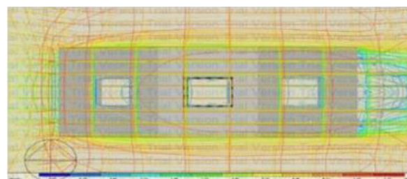
تصویر ۶- الگوی جریان هوا در اطراف ساختمان در حیاط میانی ۳ (CFD).
